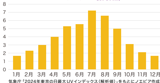
UVインデックス（解析値）*
